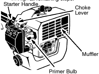
Primer Bulb
